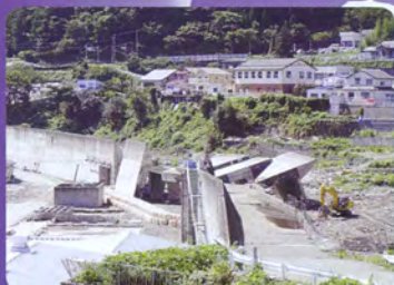
津波により破壊された唐丹湾小白浜漁港の防潮堤
